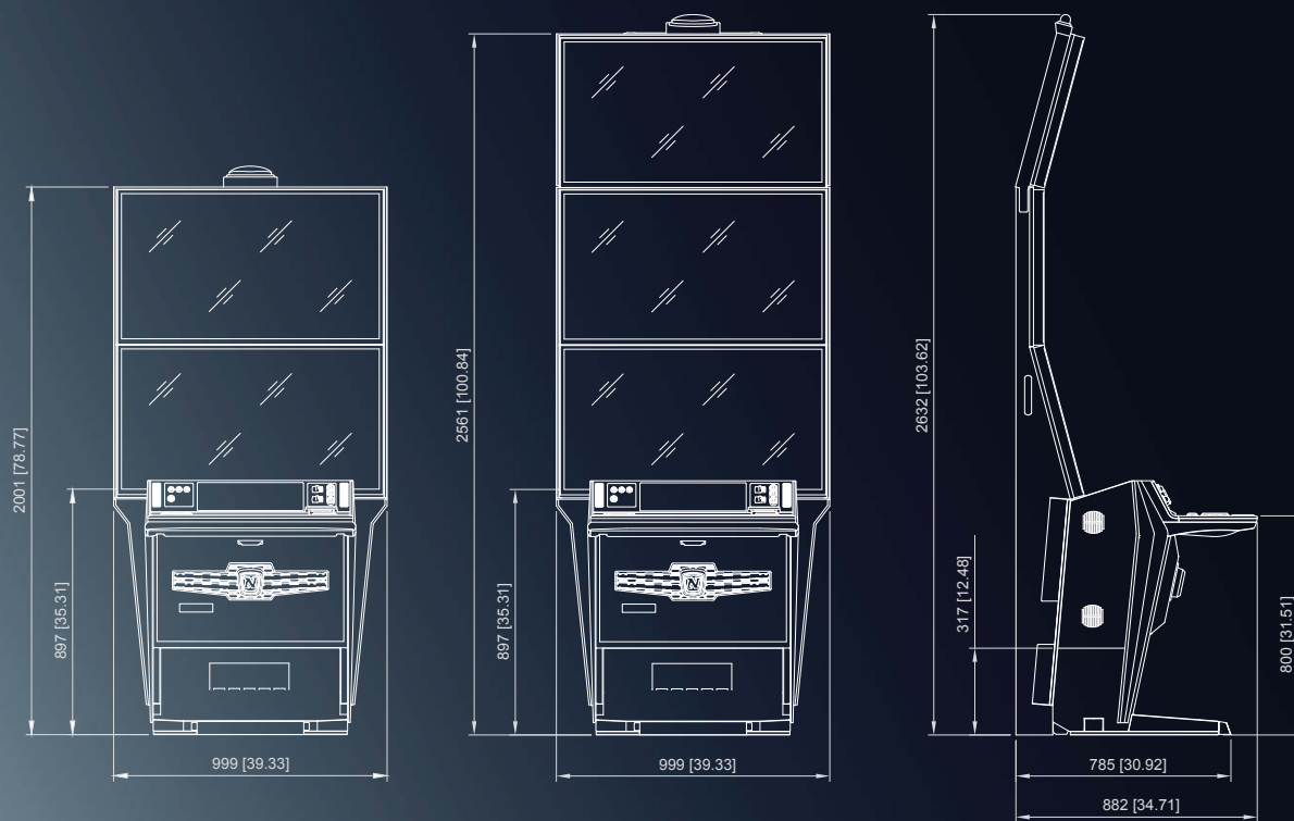
V.I.P. X Dream™ 2.43 / 3.43 (FV330D)
